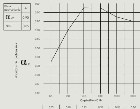
40 mm fade® PLUS+ - Montaż bezpośredni (typ A)
