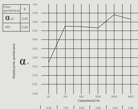
25 mm fade® PLUS+ - Montaż podwieszony (E-200)
